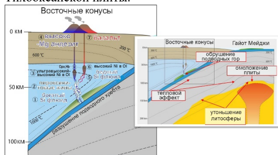
Рис. 2 – Поперечное сечение северной части зоны субдукции Камчатки и схематическая модель формирования лав ВК.
