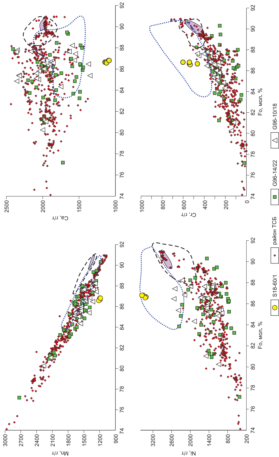
Рис. 4. Содержание Ni, Mn, Ca и Cr относительно Fo во вкрапленниках оливина из толеитов ТСБ.
