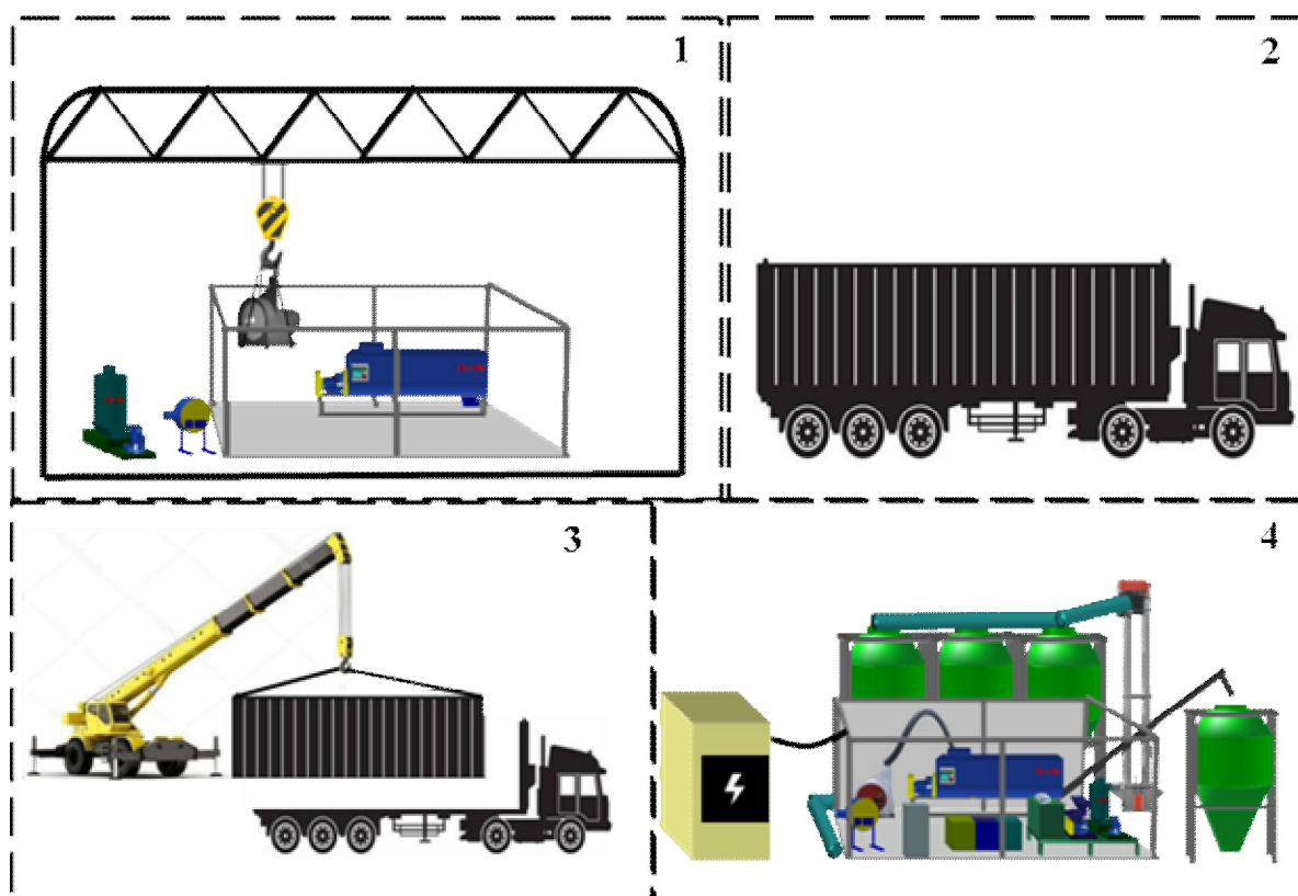
Рисунок 2 – Сборка технологического модуля на базе конструктивного модуля с габаритами грузового контейнера:
