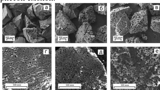
Рисунок 1 – СЭМ изображения РФ-смол; а, б, в – РФС-и, РФС-10% (CaCO 3 ), РФС-25% (CaCO 3 ), в, г, д - РФС-25% (толуол), РФС-35% (толуол), РФС-65% (толуол)
