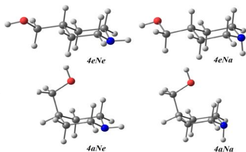
Рис. 1. Оптимизированные структуры конформеров 4-пиперидинметанола
