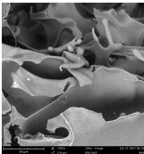
Рис.1. Микрофотография СЭМ биополимерных матриц на основе БСА
