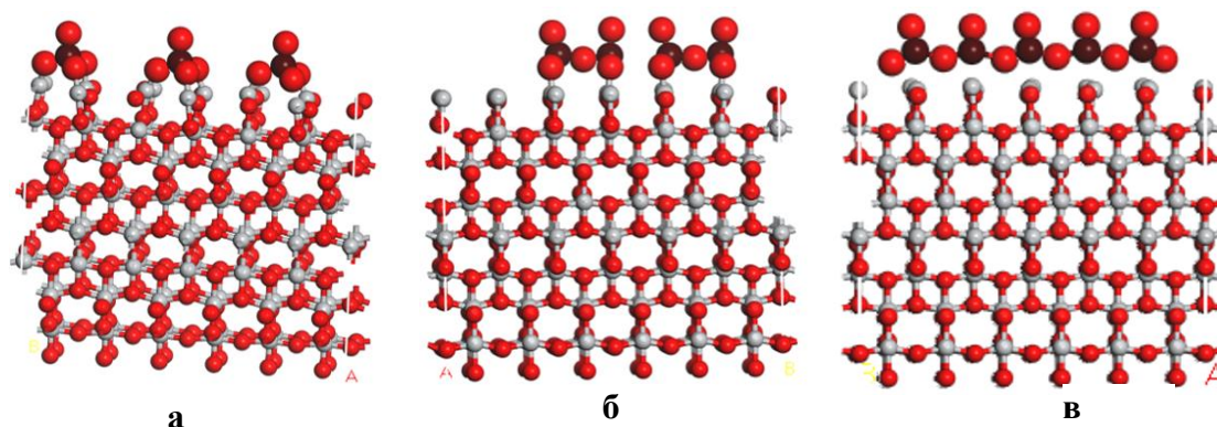
Рис. 2. Молекулярные системы изолированных (а), димерных (б) и полимерных (в) \text{VO}_x частиц на \text{TiO}_2 (анатаз).
