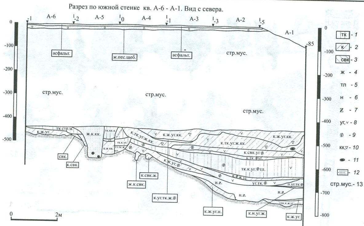
Рис. 5. Разрез заполнения восточного отрога Резницкого оврага по южной стенке раскопа Ленина-15. 1 - темно-коричневая супесь; 2 - коричневая супесь; 3 - светло-коричневая супесь; 4 - желтый суглинок; 5 - тлен; 6 - навоз; 7 - щепы; 8 - уголь; 9 - печина; 10 - кирпичная крошка; 11 - бревна; 12 - песок; 13 - строительный мусор XX в.
