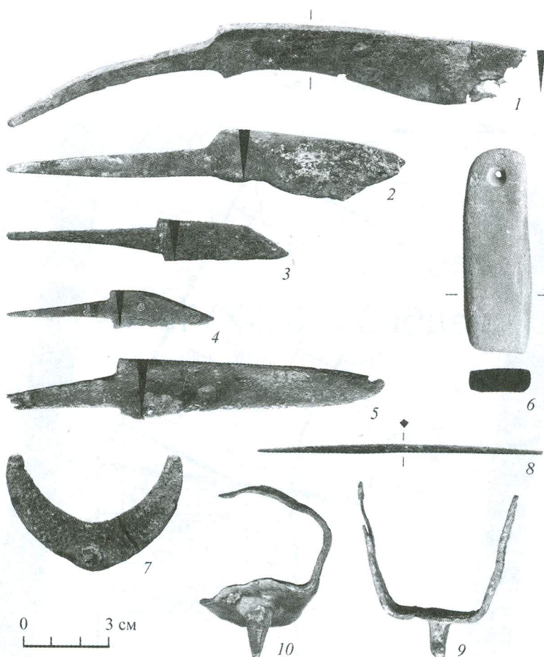
Рис. 3. Великий Новгород 2011. Раскоп Досланский. Находки из слоев XIV–XV вв. 1–4 — ножи сапожные (Досл-1-26; Досл-11-11; Досл-1-134; Досл-11-27); 5 — нож (Досл-11-16); 6 — оселок (Досл-12-2); 7 — подковка сапожная врезная с шипом (Досл-2-61); 8 — шило (Досл-12-25); 9–10 — шипы ледоходные сапожные (Досл-2-69; Досл-11-15). (1–5, 7–10 — железо; 6 — камень)
