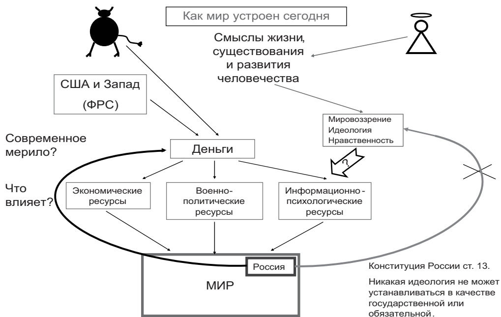
Рис. 1. Устройство мира
