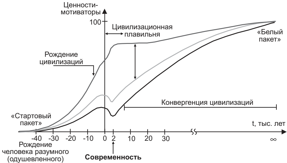
Рис. 25. Эволюция человечества
