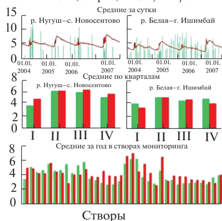
Рис. 1. Схематическое представление структуры гидрохимического блока модели, расположения пунктов гидрохимического мониторинга и видов представления расчетной гидрохимической информации.
