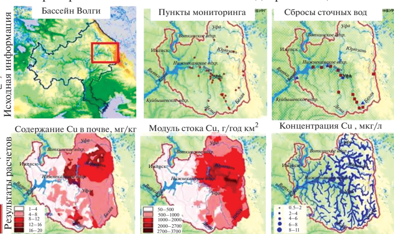
Рис. 1. Схематическое представление структуры гидрохимического блока модели, расположения пунктов гидрохимического мониторинга и видов представления расчетной гидрохимической информации.
