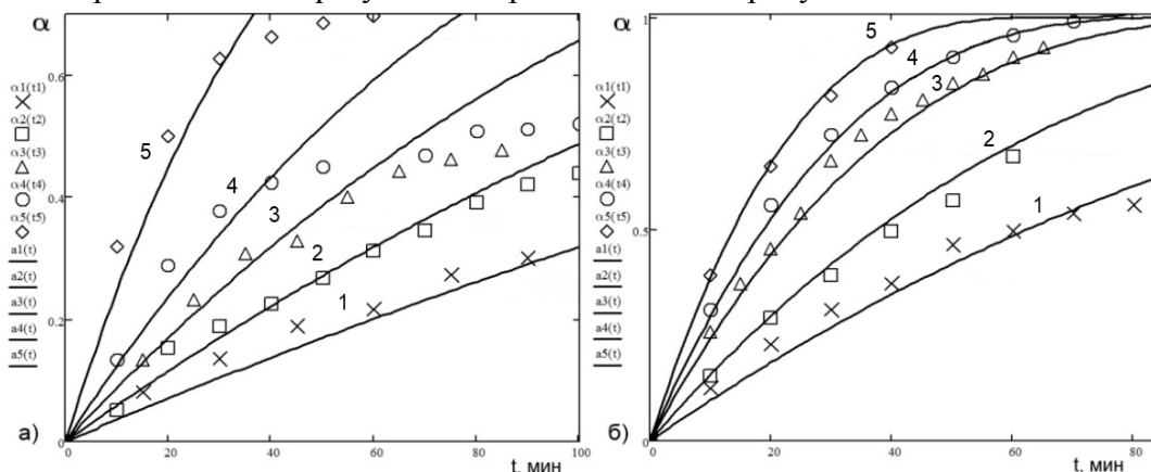
Рис. 1. Зависимость доли растворенного марганца и железа в серной кислоте от времени: а) марганец; б) железо. Точки – экспериментальные данные, линии – модельные кривые \alpha - t (модель сжимающейся сферы). Концентрация H_2SO_4 : 1 – 2.52 моль/л, 2 – 5.23 моль/л, 3 – 7.15 моль/л, 4 – 10.05 моль/л, 5 – 18 моль/л.
