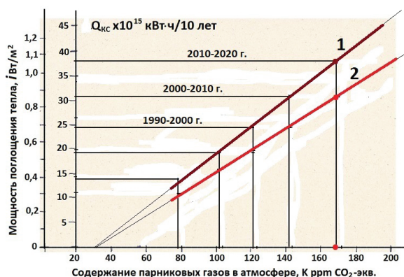
Рис. 2. Изменение количества накопленной тепловой энергии в КС Земли в каждом последующем 10-лети (1) и мощности поглощения тепла (2) в зависимости от содержания в атмосфере антропогенных ПГ
