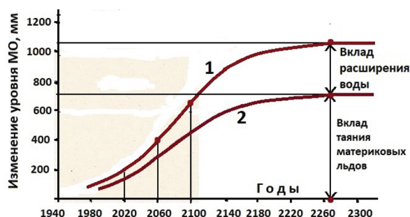
Рис. 3. Графики подъема уровня моря за счет таяния материковых льдов (2), а также общего подъема уровня (1) до момента достижения климатической системой радиационно-равновесного состояния
