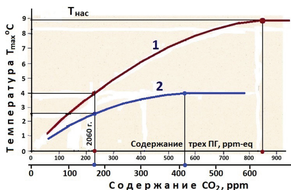
Рис. 5. График зависимости радиационно-равновесной температуры атмосферы от содержания в ней антропогенных выбросов ПГ: 1 — для выбросов трех основных парниковых газов; 2 — для выбросов диоксида углерода
