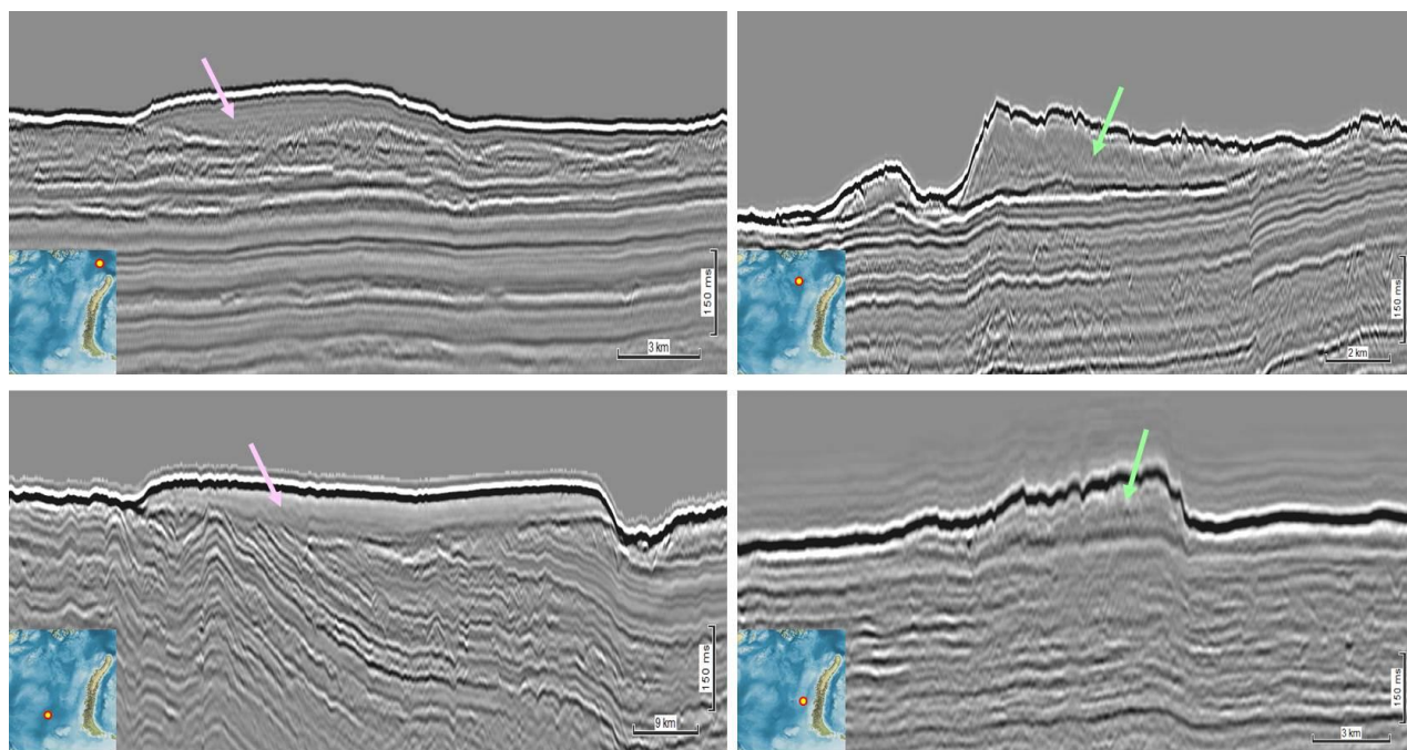
Рис. 2. «Мягкие морены» (указаны розовыми стрелками) и призмы зоны отлегания ледника (указаны зелёными стрелками) по данным 2D CP (материалы ПАО «НК «Роснефть»).
