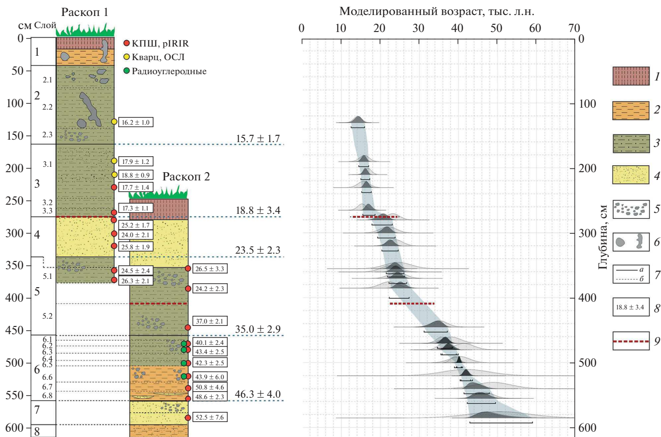
Рис. 3. Структура разреза стоянки Ушбулак, результаты абсолютного датирования и байесовского моделирования. 1 — тяжелый суглинок; 2 — суглинок; 3 — супесь; 4 — песок; 5 — гравий; 6 — кротовины; 7 — границы ( a — четкие, b — нечеткие); 8 — моделированный возраст границ, тыс. л. н.; 9 — hiatus.
