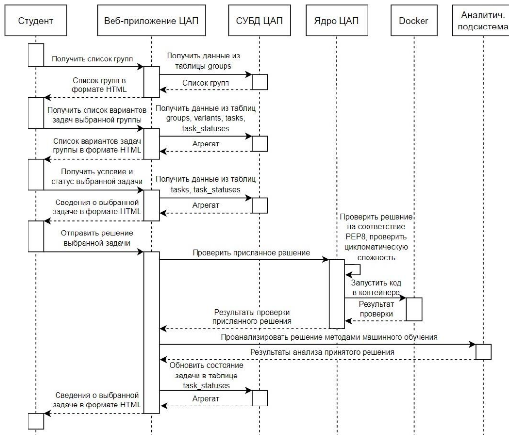
Рисунок 2. Диаграмма последовательностей системы «Цифровой ассистент преподавателя».
