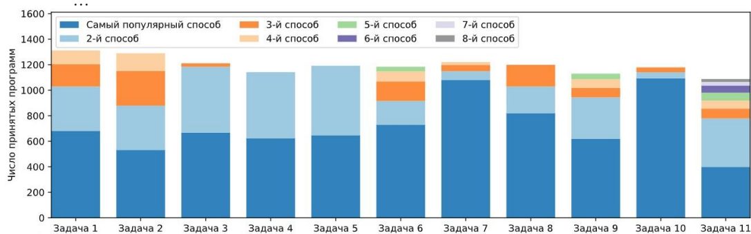
Рисунок 11. Популярность способов решения задач в зависимости от типа задачи.
