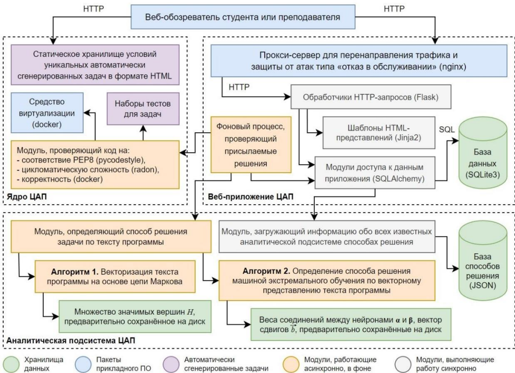
Рисунок 1. Архитектура системы Цифровой ассистент преподавателя.
