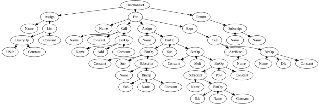
Рисунок 6. Дерево абстрактного синтаксиса для одного из решений уникальной задачи, относящихся к типу 4 (см. таблицу 1), построенное при помощи стандартной библиотеки Python.
