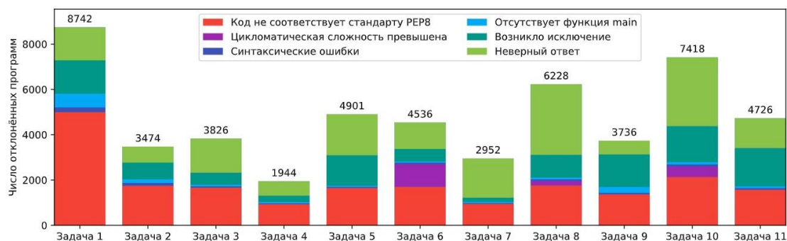
Рисунок 10. Причины отклонений присланных студентами решений в зависимости от типа задачи.
