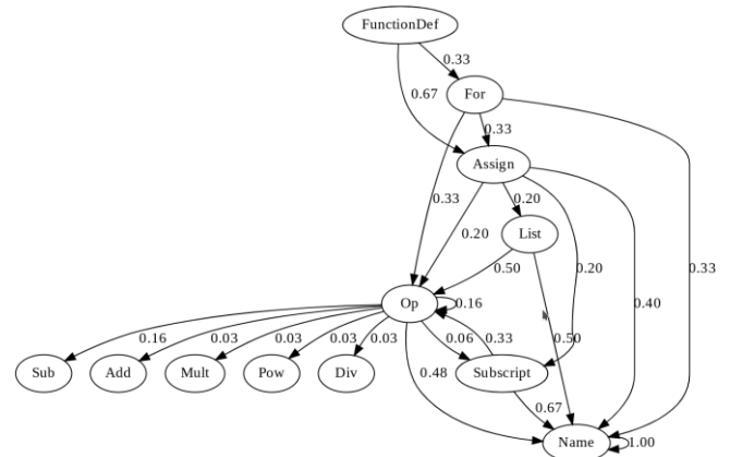
Рисунок 7. Граф переходов между состояниями цепи Маркова для дерева абстрактного синтаксиса, показанного на рис. 6.
