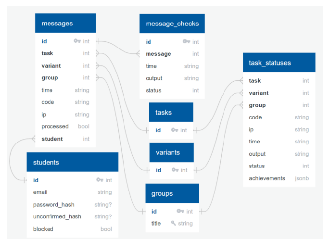
Рисунок 3. Диаграмма сущность-связь базы данных веб-приложения Цифровой ассистент преподавателя.
