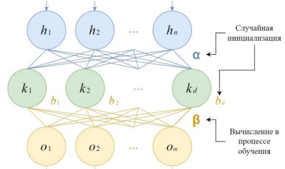
Рисунок 8. Машина экстремального обучения.
