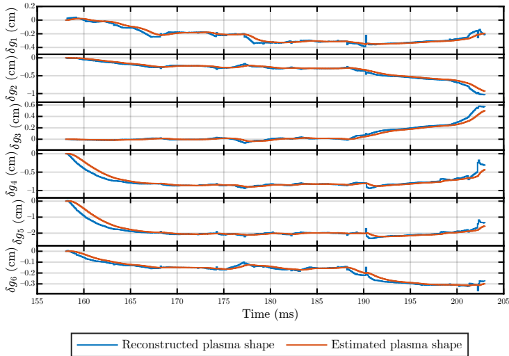
Рисунок 12 — Сравнение вариаций зазоров \delta g на выходе LPV-модели, вычисленной по восстановленному алгоритмом FCDI-IT равновесию (синяя линия), и оценки вариаций зазоров \delta \tilde{g} , полученных с помощью робастного наблюдателя (красная линия). Разряд № 37263 токамака Глобус-М2.
