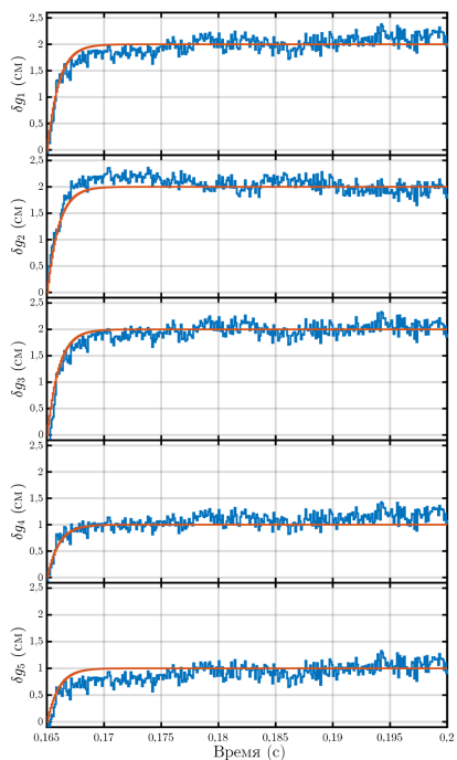
Рисунок 9 — Результаты полунатурного моделирования системы управления ударными точками g_{1-2} и зазорами g_{3-5} во время диверторной фазы разряда № 37326 токамака Глобус-М2. Красные линии - задающие воздействия.
