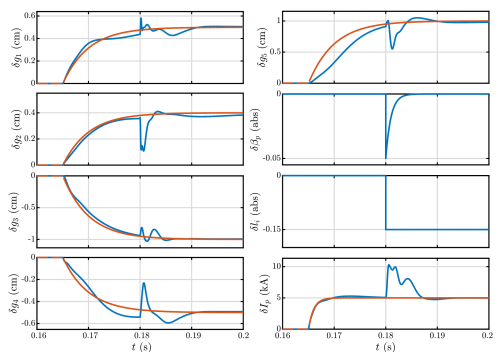
Рисунок 14 — Результаты моделирования системы магнитного управления плазмой с внутренним каскадом управления по потокам на магнитных петлях на модели разряда №37239 токамака Глобус-М2. Красным обозначены задающие воздействия.
