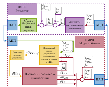
Рисунок 10 — Структурная схема системы магнитного управления плазмой для токамака Глобус-М2 при полунатурном моделировании.
