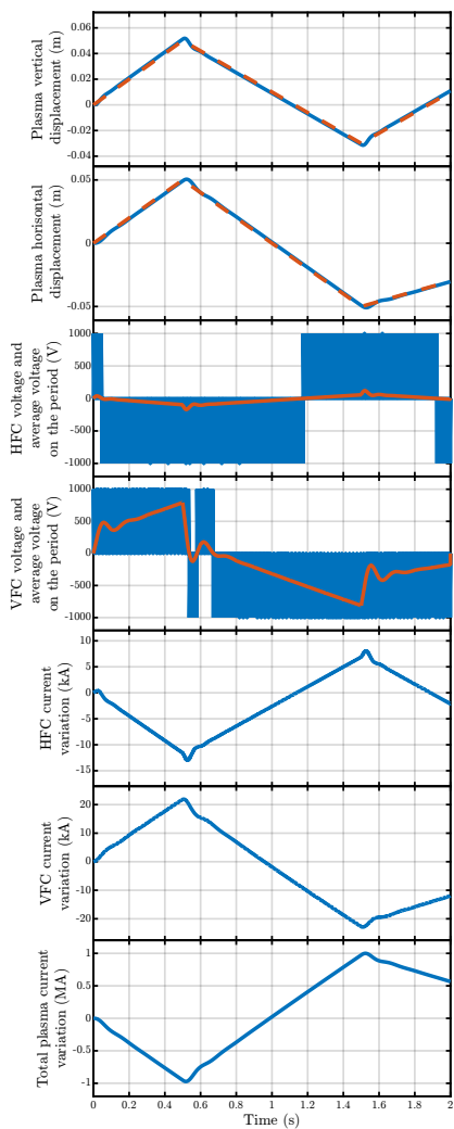
Рисунок 8 — Результаты моделирования системы управления положением плазмы в токамаке ИГНИТОР, напряжения на ОГУП и ОВУП и их средние за период ШИМ, которые показаны красными линиями, смещения токов в ОГУП и ОВУП и отклонение тока плазмы. Красные пунктирные линии являются задающими воздействиями.
