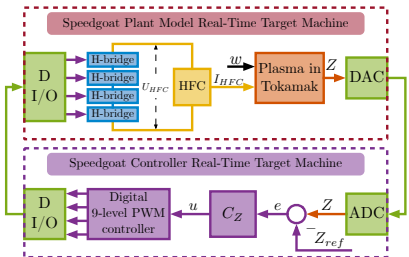
Рисунок 6 — Структурная схема системы управления с инвертором напряжения в режиме 9-уровневой ШИМ при проведении полунатурного моделирования.
