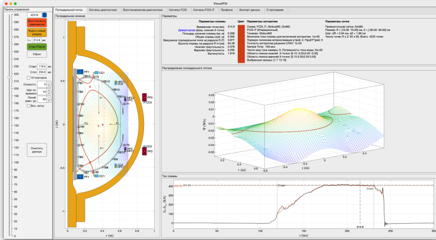
Рисунок 11 — VisualPSI отображает равновесие плазмы в течение разряда № 42416 токамака Глобус-М2, восстановленное алгоритмом FCDI-IT.
