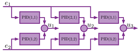
Рисунок 1 — Пример матричного ПИД-регулятора с двумя входами ( e_1, e_2 ) и тремя выходами ( u_1, u_2, u_3 ).
