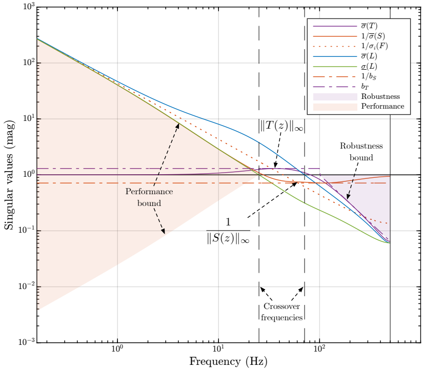
Рисунок 3 — Пример, иллюстрирующий метод синтеза. Сингулярные значения частотных откликов передаточных функций L(z) , S(z) и T(z) многомерной цифровой системы управления и функции формы ( b_S , b_T ).
