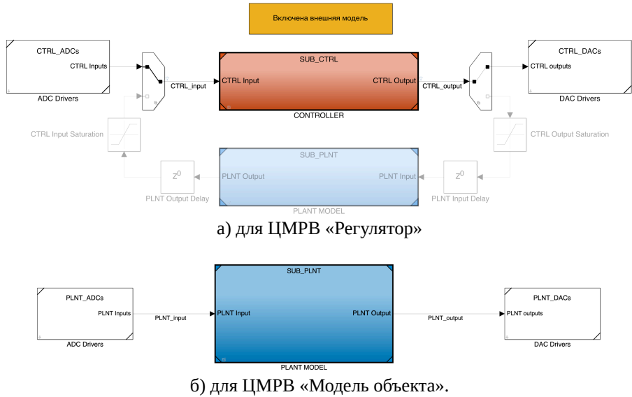
Рисунок 5 — Simulink-схемы верхнего уровня.
