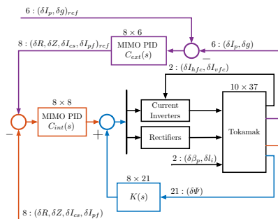
Рисунок 13 — Структурная схема системы управления формой плазмы с внутренним каскадом управления по потокам на магнитных петлях (выделен синим).
