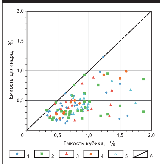
Рис. 7. СРАВНЕНИЕ ЕМКОСТИ КУБИКОВ (5×5 см) И ЦИЛИНДРОВ (3×3 см) РИФЕЙСКИХ ОТЛОЖЕНИЙ ЮРБУЧЕНО-ТОХОМСКОГО МЕСТОРОЖДЕНИЯ
