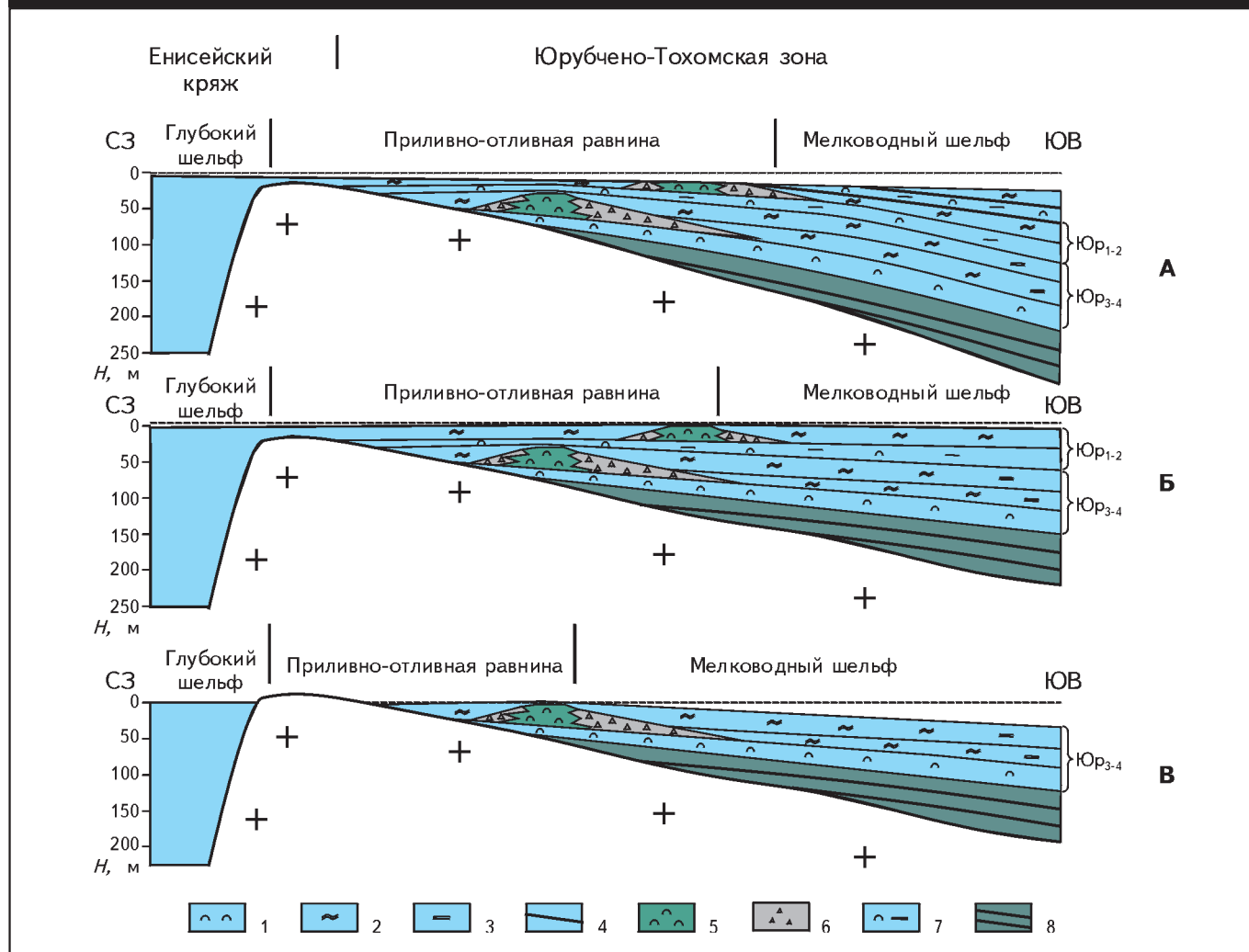
Рис. 1. МОДЕЛЬ ОСАДКОНАКОПЛЕНИЯ РИФЕЙСКИХ ОТЛОЖЕНИЙ ЮРУБЧЕНО-ТОХОМСКОЙ ЗОНЫ
