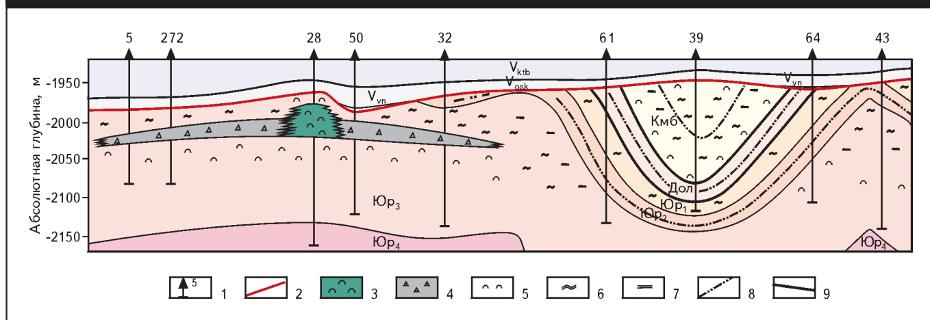
Рис. 2. ПРИНЦИПИАЛЬНАЯ МОДЕЛЬ ФОРМИРОВАНИЯ ЮРУБЧЕНСКИХ ОТЛОЖЕНИЙ ЮРУБЧЕНО-ТОХОМСКОГО МЕСТОРОЖДЕНИЯ
