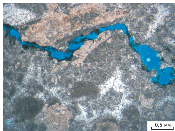
Рис. 5. ОТКРЫТАЯ СТИЛОЛИТОПОДОБНАЯ ТРЕЩИНА С ПУСТОТАМИ ВЫЩЕЛАЧИВАНИЯ В ОБЛОМОЧНОМ ОКРЕМНЕННОМ ДОЛОМИТЕ
