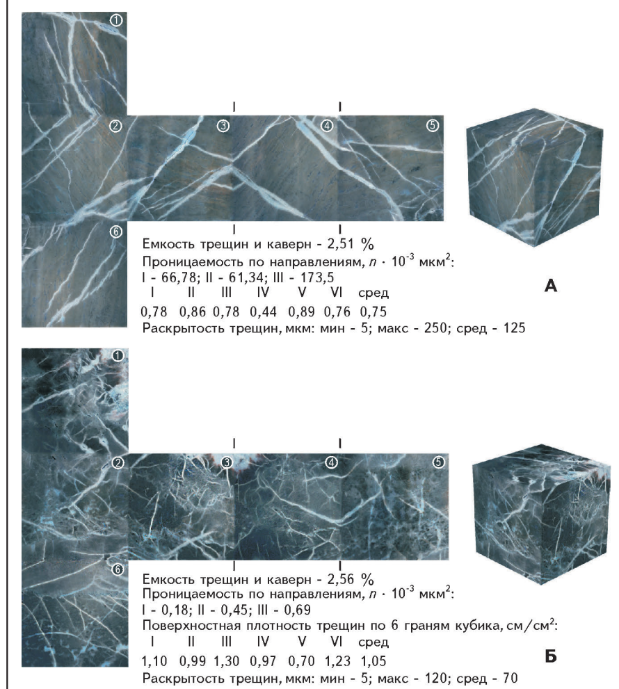
Рис. 11. НЕОДИНАКОВОЕ ВЛИЯНИЕ ТРЕЩИНОВАТОСТИ НА ФИЛЬТРАЦИЮ УВ (Юрубчено-Тохомское месторождение)
