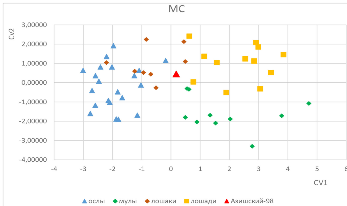
Рис. 4. Положение экземпляра из погребения 1 кургана «Азишский-98» среди лошадей, ослы и их гибридов в пространстве первых двух канонических переменных по результатам дискриминантного анализа измерений кости пясти.
