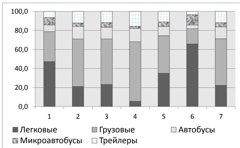
Рисунок 2 Вклад каждой категории транспорта в суммарный выброс загрязнителей, % (Примечание: На диаграмме цифрами обозначены 1 - CO, 2 - NO2, 3 - углеводороды, 4 - сажа, 5 - SO2, 6 - формальдегид, 7 - бенз(а)пирен)
